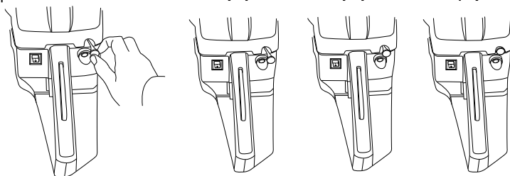
рычаг заслонки
