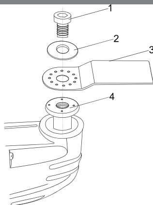
Установка ножа
